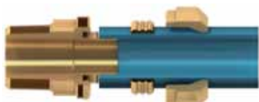
Aansluitkoppeling 66 serie buitendiameter t/m 75 mm
